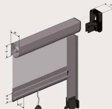
Maniglia con cricchetto
