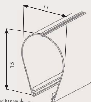
Dimensioni cassonetto e guida
