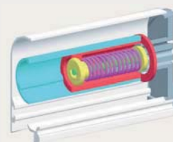
Sistema light, freno per molla
