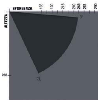
Lunghezza del braccio e inclinazione Installazione a parete
