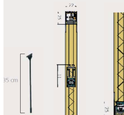
Sezione Verticale e Astina di movimento
