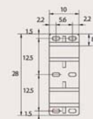
Supporto a parete
