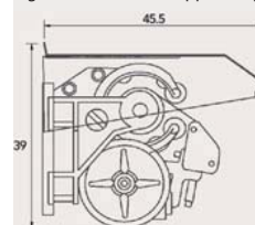
Ingombro tenda con tettuccio in alluminio estruso
