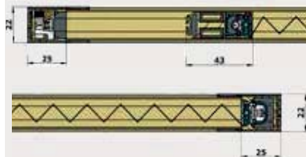
Sezione Verticale
