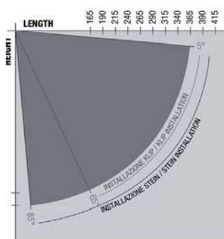
Lunghezza del braccio e inclinazione Installazione a parete o soffitto
