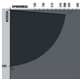
Lunghezza del braccio e inclinazione Installazione a soffitto
