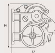
Ingombro tenda con supporto a parete
